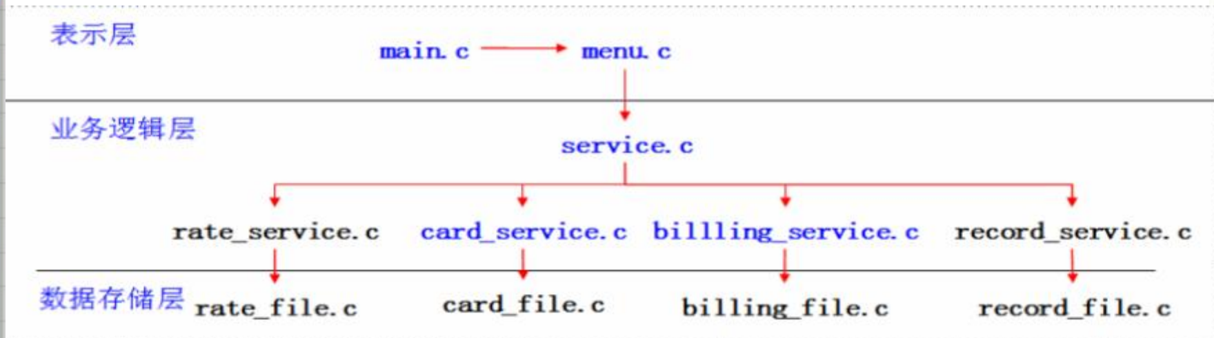
图 2.2 系统层次设计图
